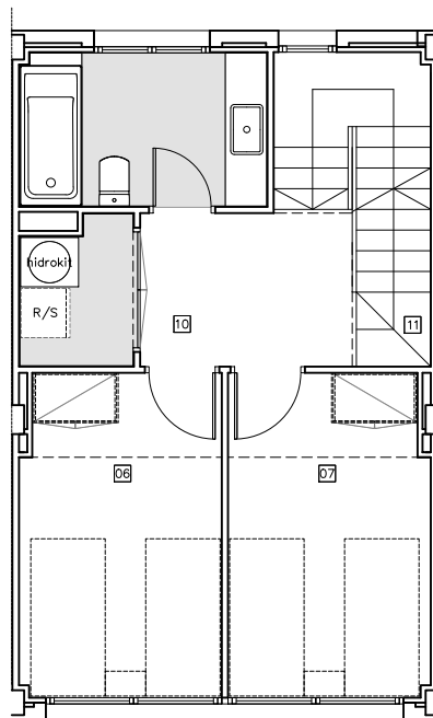
PLANTA PRIMERA HABITATGE 2
