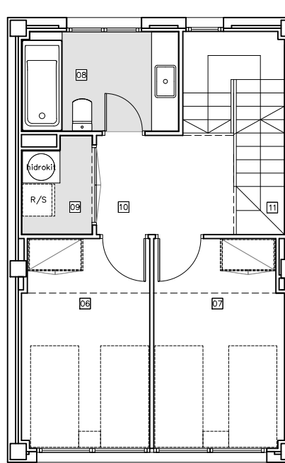
PLANTA PRIMERA HABITATGE 1
