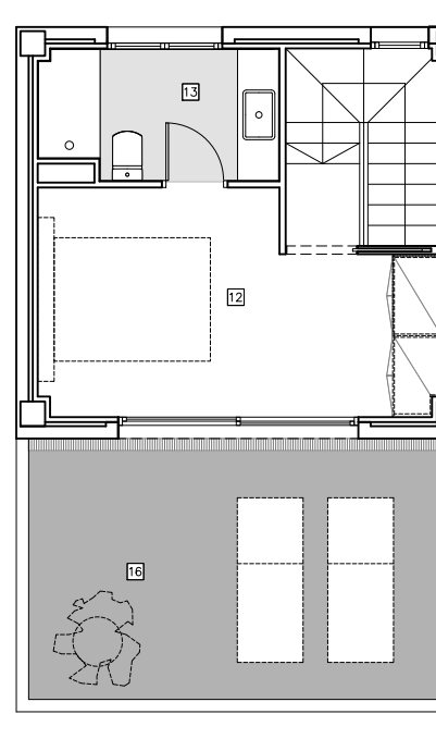
PLANTA SEGONA HABITATGE 1
