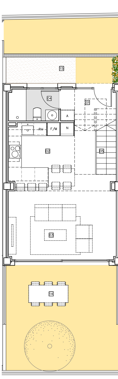
PLANTA BAIXA HABITATGE 1
