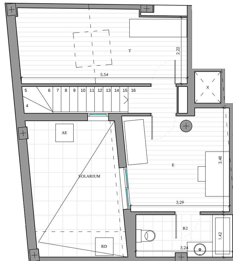
C/ SANT PERE 4-6 Tercer primera (planta superior)
