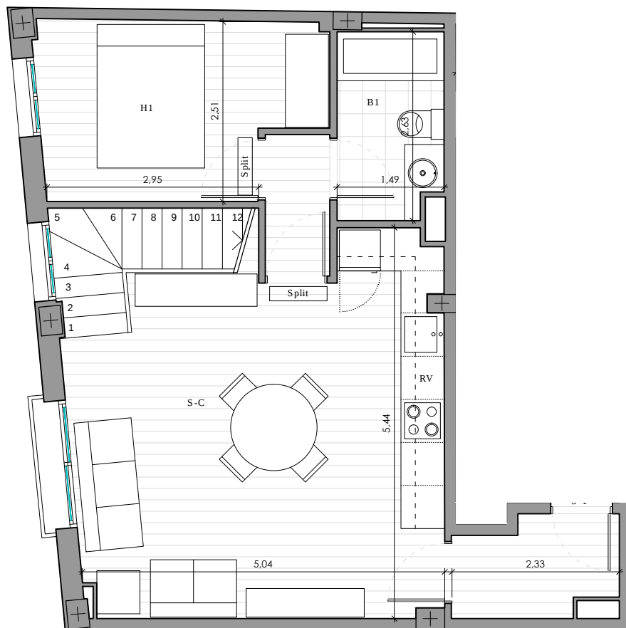
C/ SANT PERE 4-6 Tercer primera (planta inferior)
