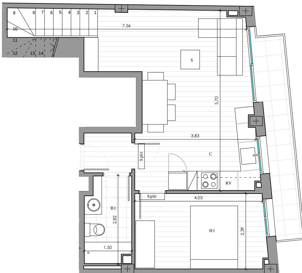
C/ SANT PERE 4-6 Tercer segona (planta inferior)
